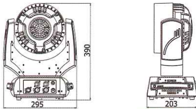
LEDWash300X 外観図
