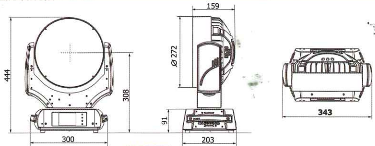
LEDWash600X 外観図
